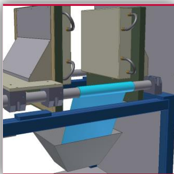
Auffangrutsche - ARH
