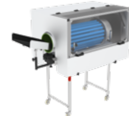
Separiertrommel mit Schallschutzhaube
