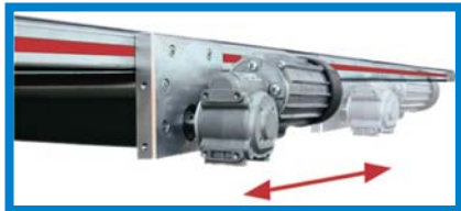
Commande d'entraînement central avec moteur à bride latérale
