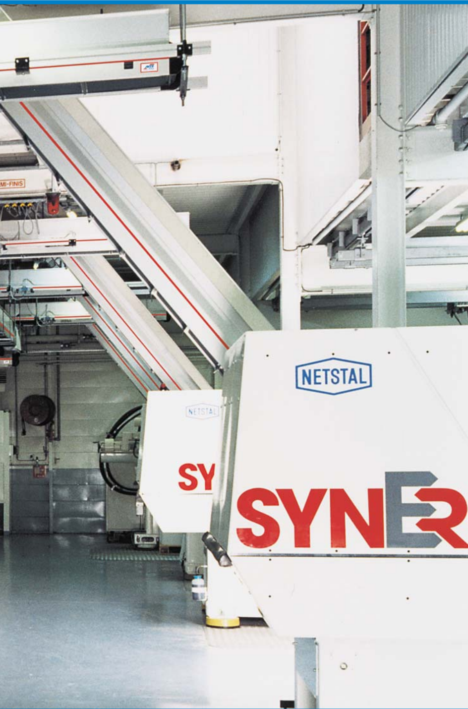
Une automatisation assistée par ordinateur entre la machine de moulage par injection et la presse: les pièces moulées par injection peuvent être distribuées aux autres convoyeurs grâce aux convoyeurs transversaux à réglage pneumatique de MTF Technik.
